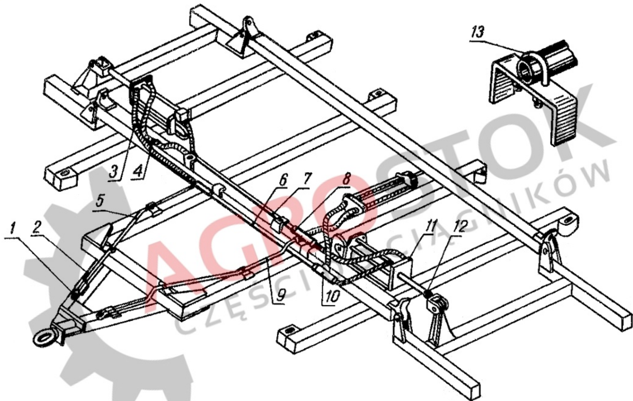
Rys.6 Instalacja hydrauliczna
