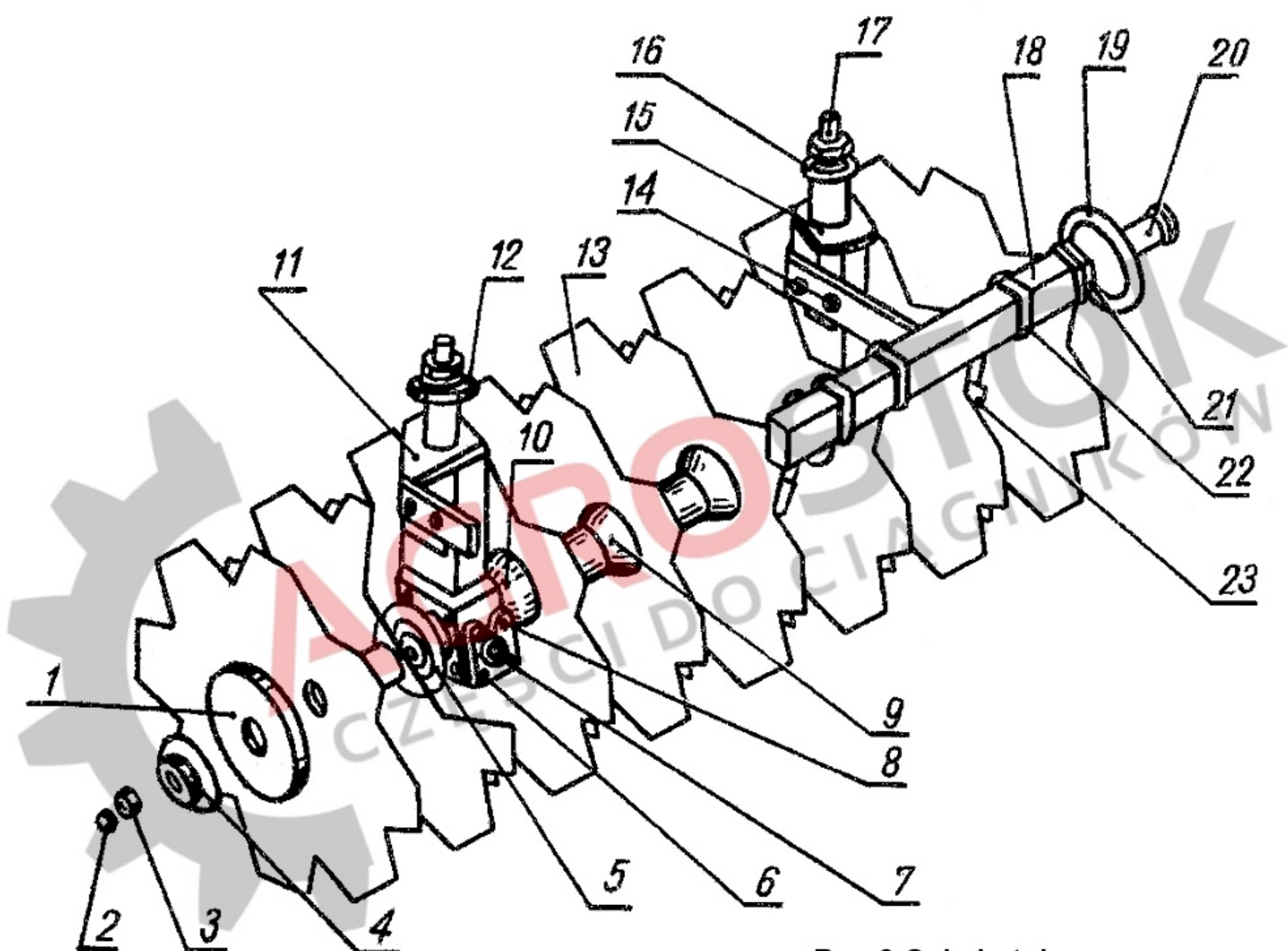
Rys.3 Sekcja talerzy
